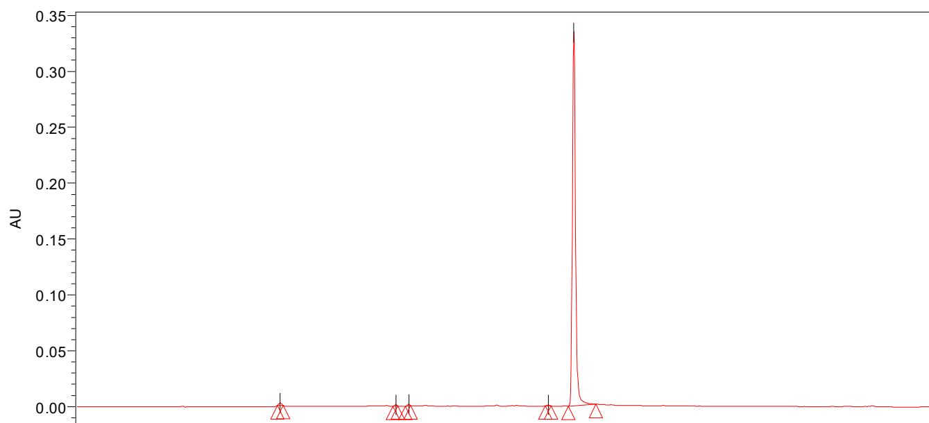
堆叠色谱图
